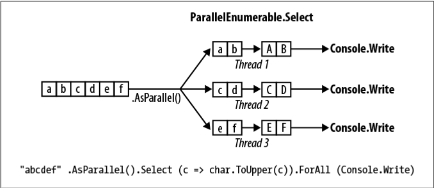
Figure 23-3. PLINQ ForAll
